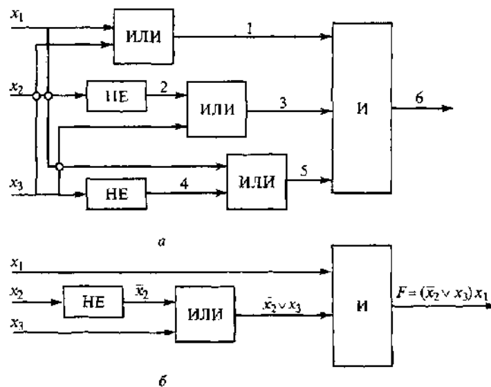
Рис. 4.8. Логические схемы булевой функции F : a - заданная схема; b - минимизированная схема
