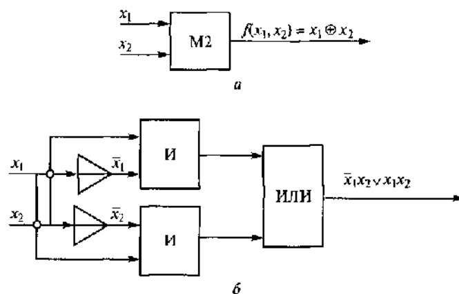
Рис. 4.15. Элемент и схема для операции M2:
