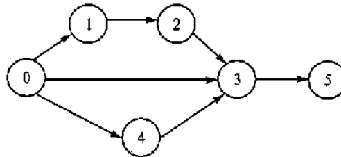
Рис. 2.20. Диаграмма последовательности работ при строительстве здания
