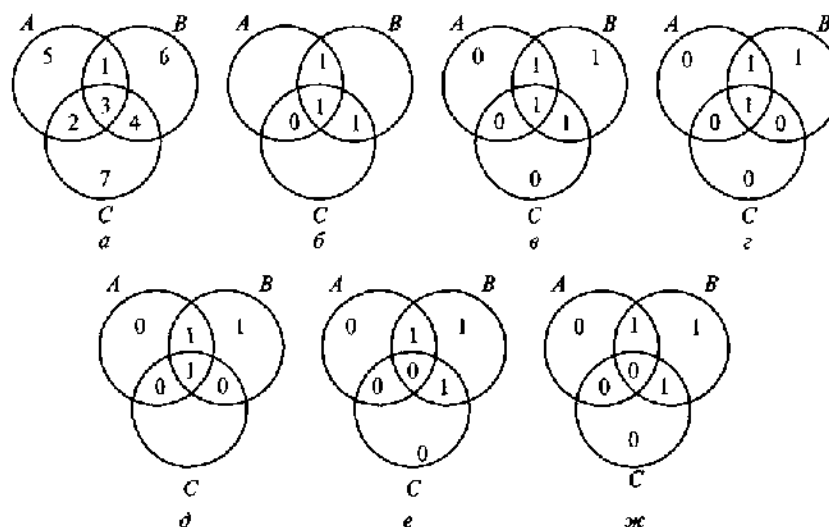
Рис. 6.9. Контроль по четности:
