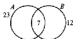
Рис. 1.21. Схематическое изображение условия задачи 15
