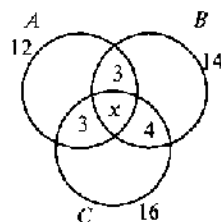
Рис. 1.22. Схематическое изображение условия задачи 16
