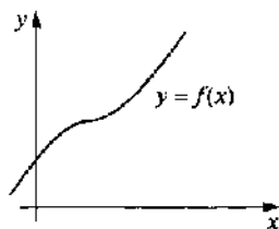
Рис. 1.6. График непрерывного биективного отображения y = f(x)
