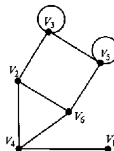
Рис. 2.19. Граф к задаче 20
