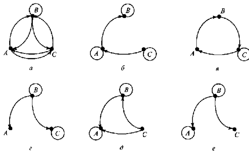
Рис. 2.29. Задание графа G к упр. 2.4 (a—e — варианты)
