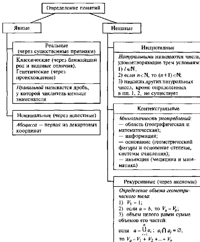
Рис. 3.8. Классификация видов определения понятий
