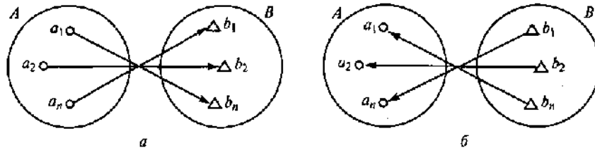
Рис. 1.7. Иллюстрация биекции:
