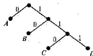
Рис. 6.2. Двоичное дерево для четырех символов
