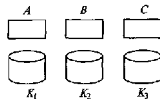
Рис. 2.7. Иллюстрация к задаче «О трех колодцах»
