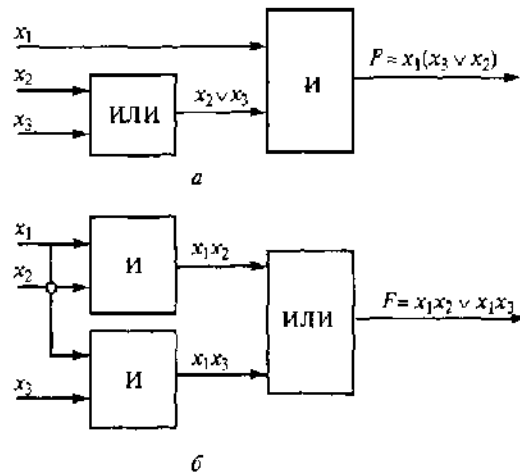
Рис. 4.7. Логическая схема булевой функции F : a - F(x_1x_2x_3) = x_1(x_2 \vee x_3) ; b - F(x_1x_2x_3) = x_1x_2 \vee x_1x_3
