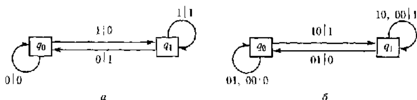
Рис. 7.4. Графы элементов памяти: а — элемент задержки; б — двухвходовый триггер
