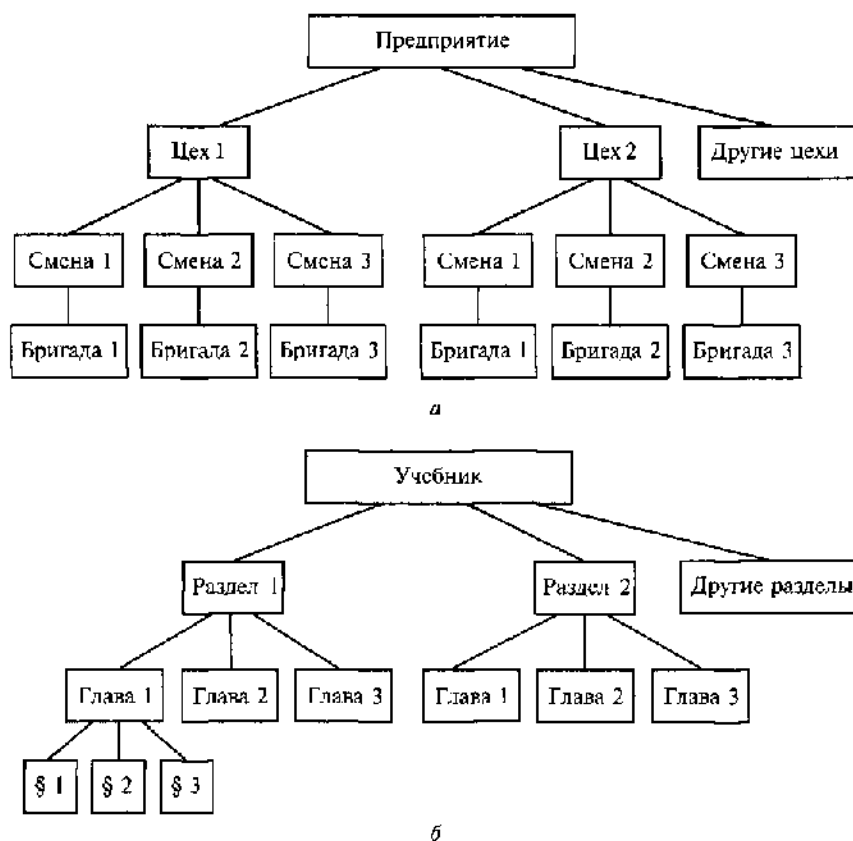
Рис. 2.23. Блок-схема иерархической структуры: а — предприятие; б — учебник
