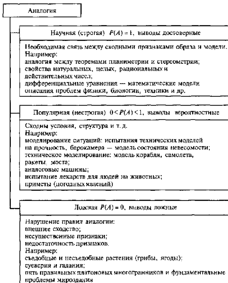
Рис. 5.13. Виды аналогии
