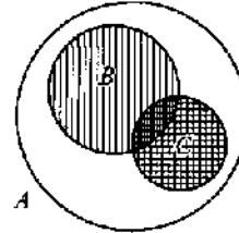
Рис. 3.2. Иллюстрация отношения между понятиями
