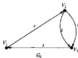
Рис. 2.3. Ориентированный граф
