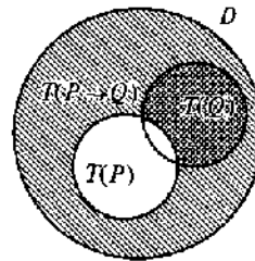
Рис. 5.5. Множество истинности импликации предикатов
