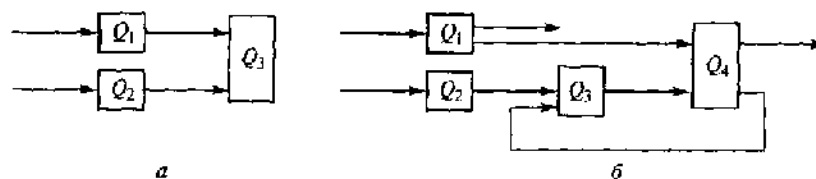
Рис. 7.3. Схема автоматов: а — простая; б — сложная
