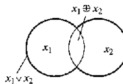
Рис. 4.14. Связь между дизъюнкцией x_1 \vee x_2 и суммой по модулю два x_1 \oplus x_2
