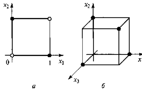
Рис. 4.16. Геометрическая интерпретация суммы по модулю два: а — на плоскости; б — в пространстве
