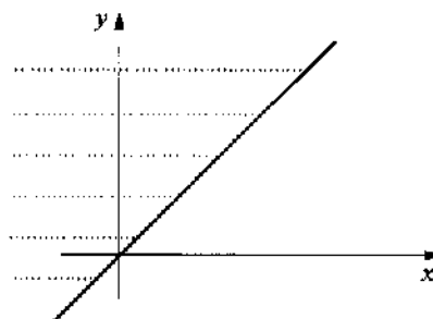
Рис. 1.15. Иллюстрация бинарного отношения R(x \leq y, \text{ где } x, y \in \mathbb{R})
