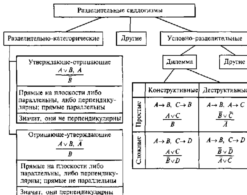
Рис. 5.9. Разделительные силлогизмы
