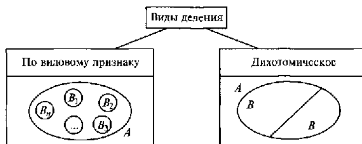
Рис. 3.9. Классификация видов деления понятий
