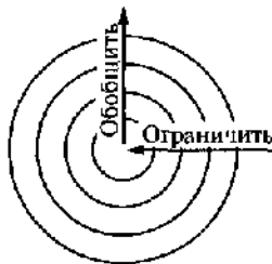
Рис. 3.3. Схема взаимно-обратных переходов ограничения и обобщения понятий
