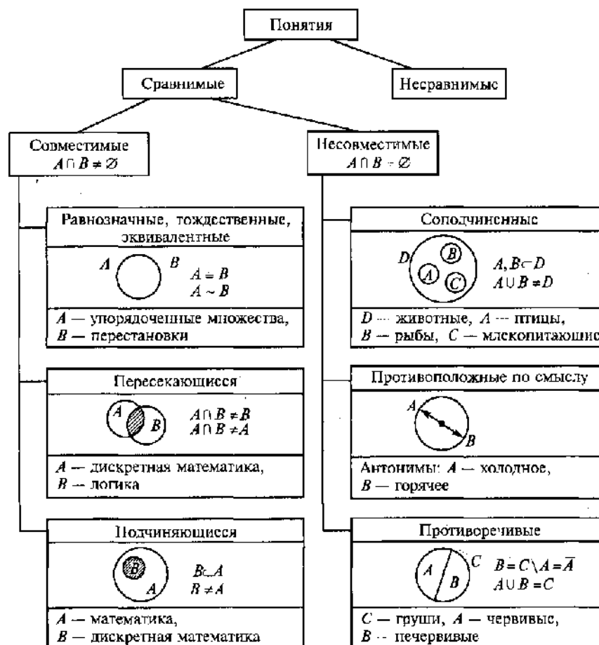
Рис. 3.5. Классификация отношений между понятиями
