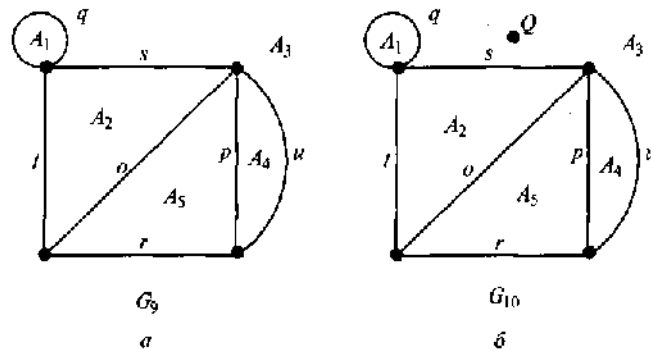
Рис. 2.6. Графы:
