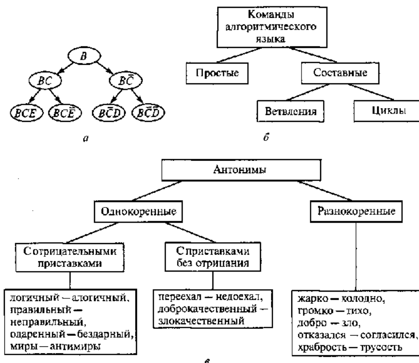
Рис. 3.10. Схема дихотомической классификации: а — бинарное дерево; б — команды алгоритмического языка; в — понятие «антонимы»
