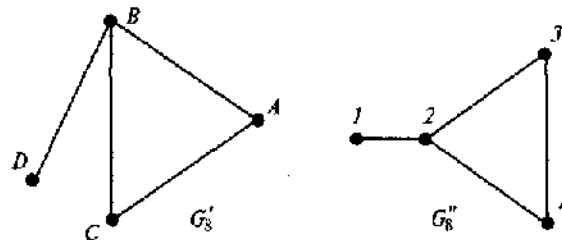
Рис. 2.5. Изоморфные графы
