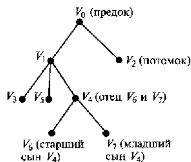
Рис. 2.15. Иллюстрация родственных связей — упорядоченное дерево
