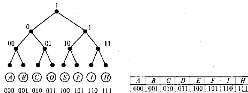
Рис. 6.1. Двоичное дерево для восьми символов.
