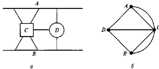
Рис. 2.11. Иллюстрации к задаче «О кёнигсбергских мостах»: а — условие; б — граф
