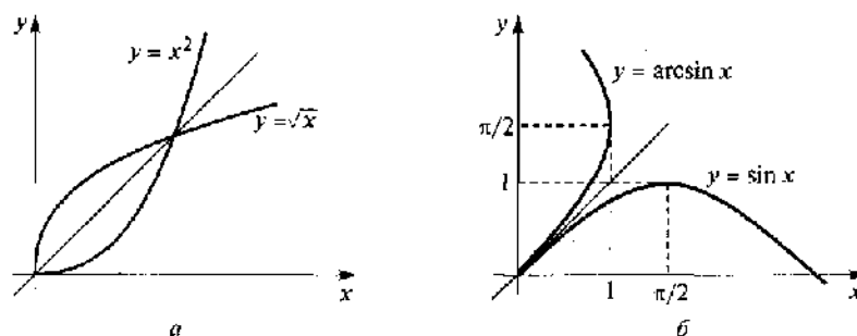
Рис. 1.16. Графики прямых и обратных бинарных отношений: a - y = \sqrt{x} и y = x^2 ; b - y = \sin x и y = \arcsin x
