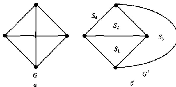
Рис. 2.8. Планарные графы:
