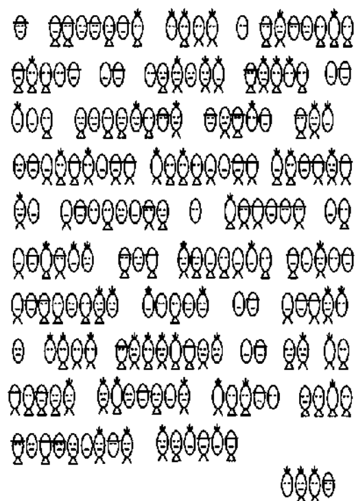
Рис. 6.10. Зашифрованное письмо
