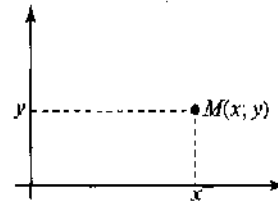
Рис. 1.3. Задание отображения xRu с помощью метода координат
